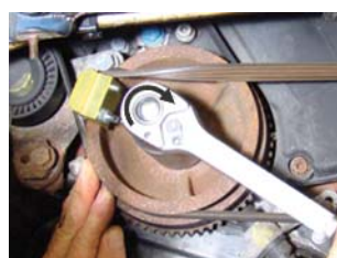
Riemen montieren
